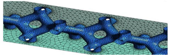
Fig. 3- Geometry of (Z. Wu et al.) [7].
